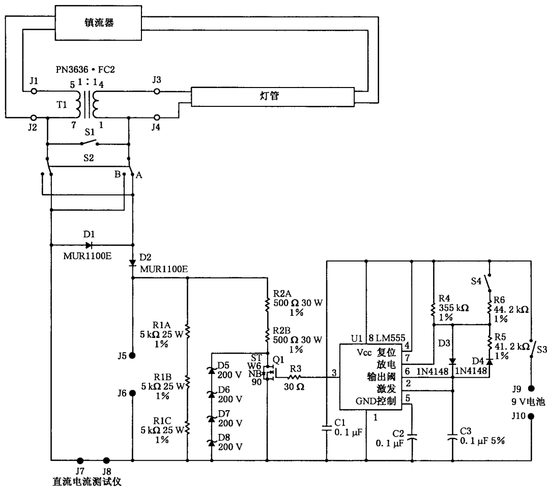
图 H. 1 不对称脉冲试验电路
