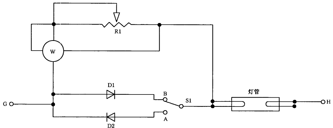
图 H.2 不对称功率试验电路
