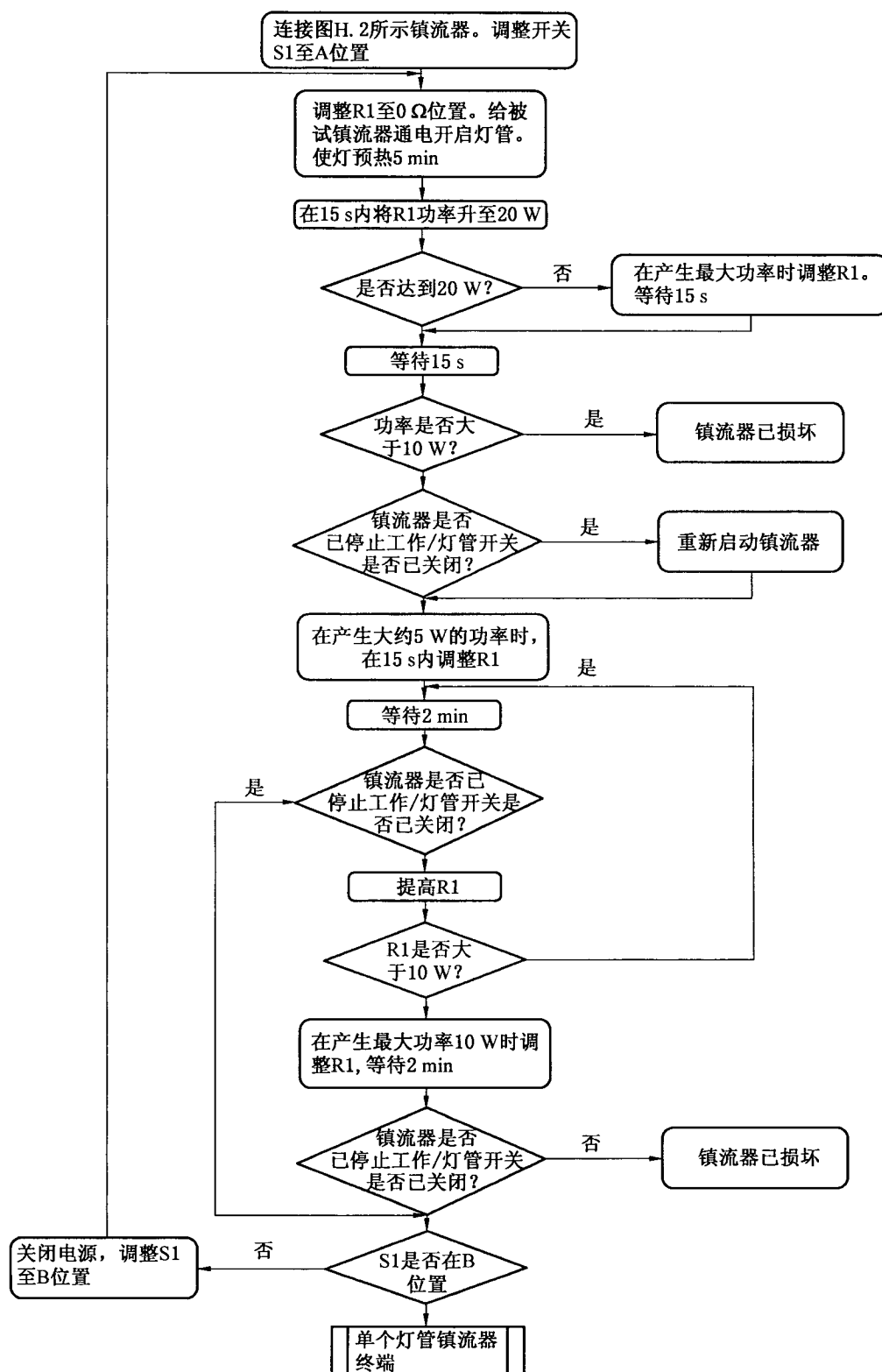
图 H.3 流程图: 不对称功率试验
