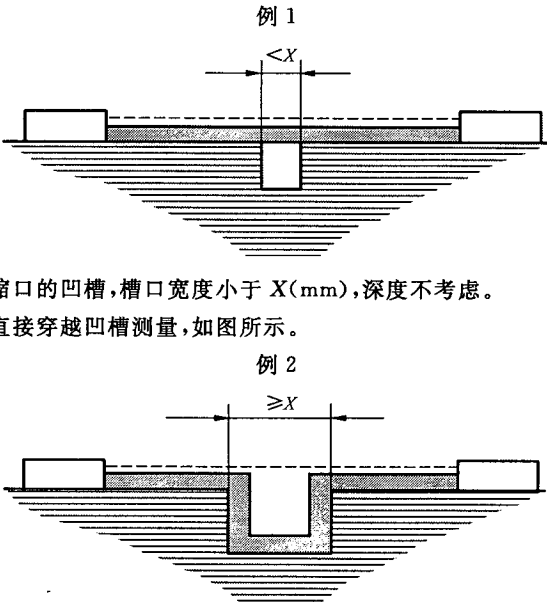
图 1 电气间隙和爬电距离的测量
