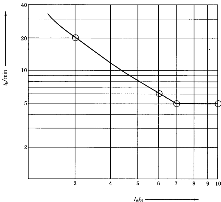
图 2 电动机 t_E 时间最小值与启动电流比 I_A/I_N 的关系
